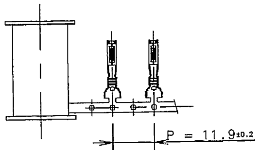
SEZ. B-B
