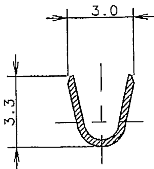
SEZ. A-A
