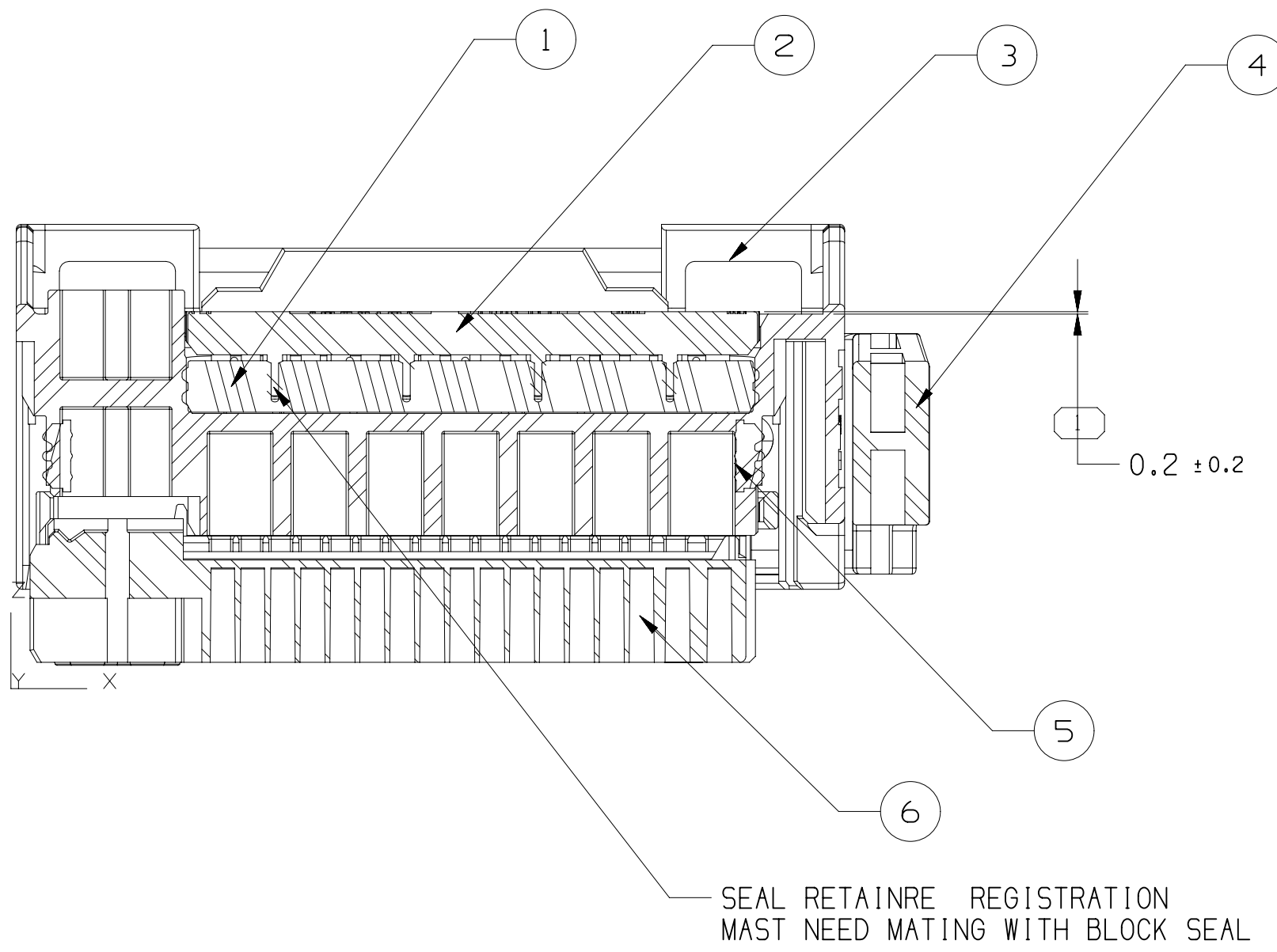
SECTION A-A
